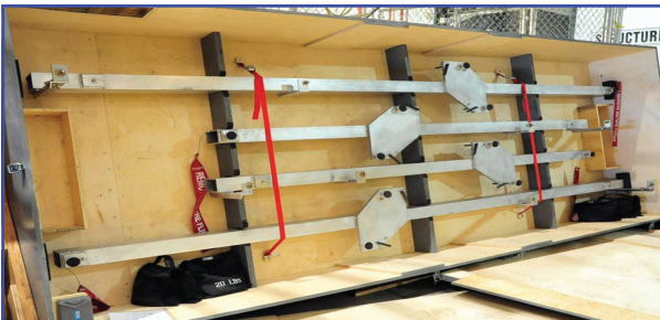
J27081-1 O/B Flap Rig
