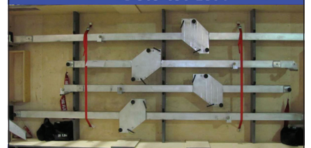
J27081-1 O/B FLAP RIG
